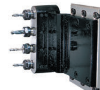
Дополнительный сверлильный суппорт
