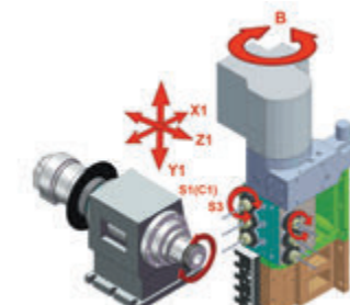
Кинематическая схема станка с осью В
